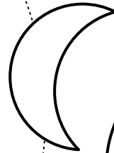
MOND
