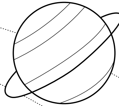
URANUS
