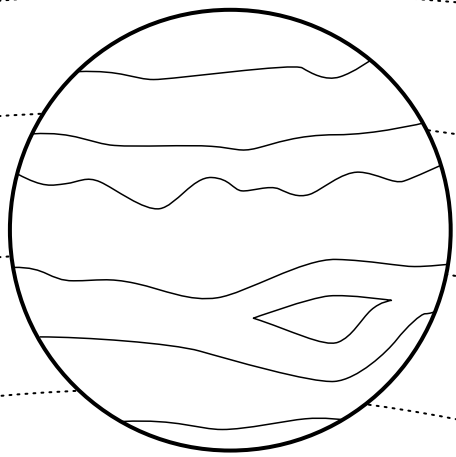
JUPITER
