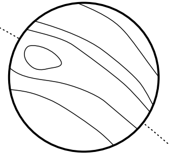
NEPTUN
