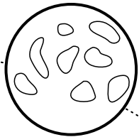
MERKUR
